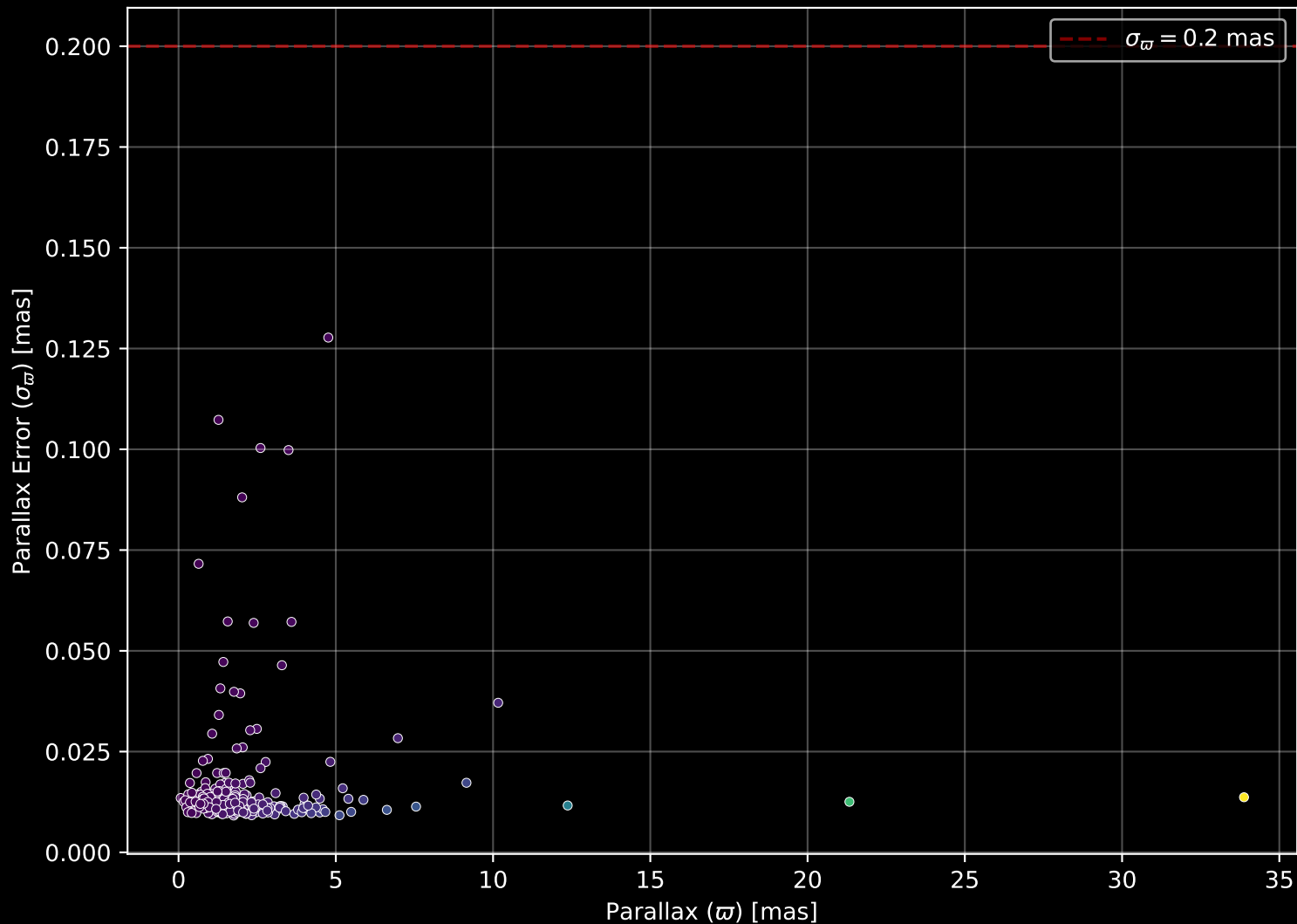
GALAH DR4 Field: [6957] Parallax Quality (n= 268)
