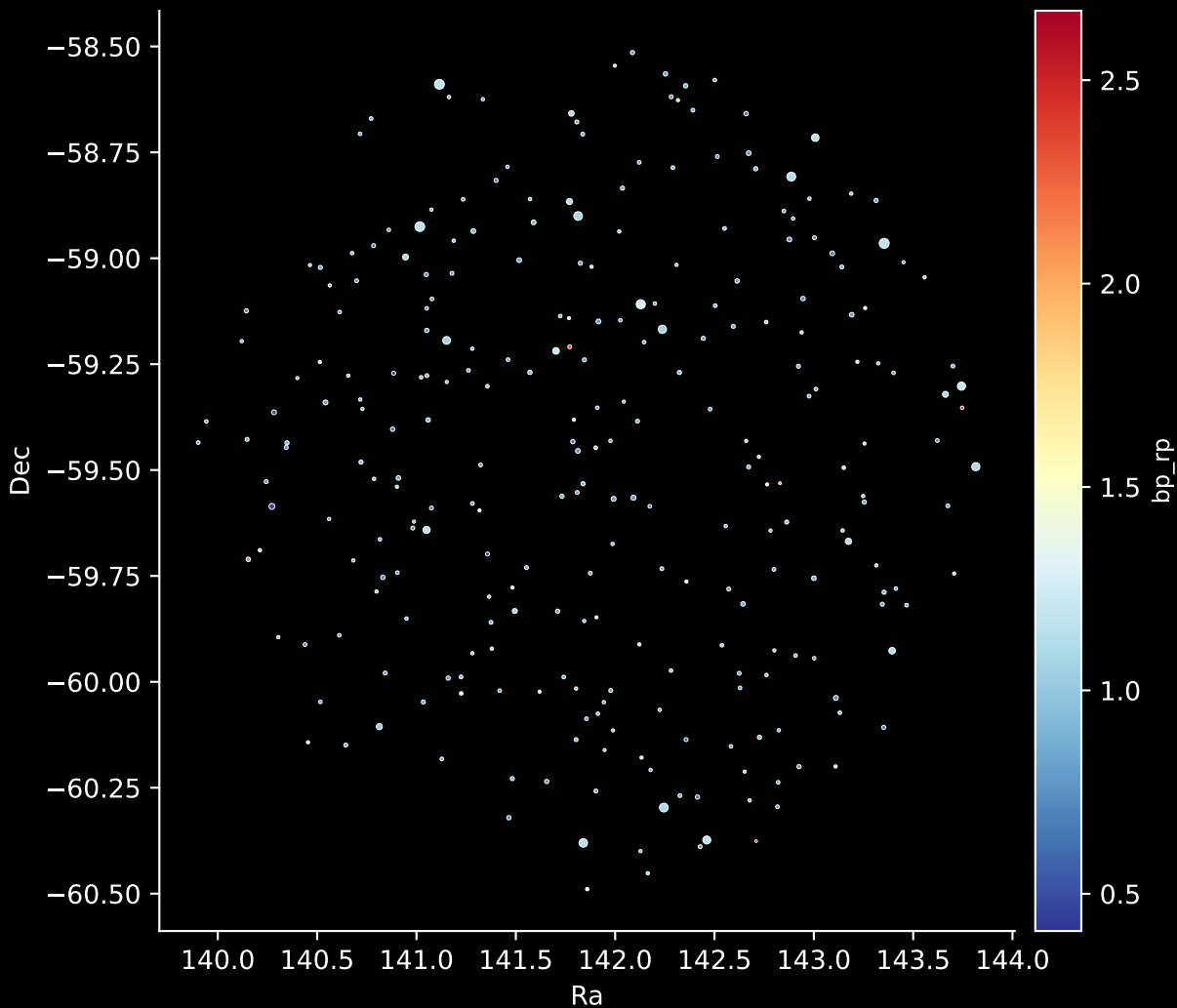
GALAH DR4 Field: [6957] Stars: 268
