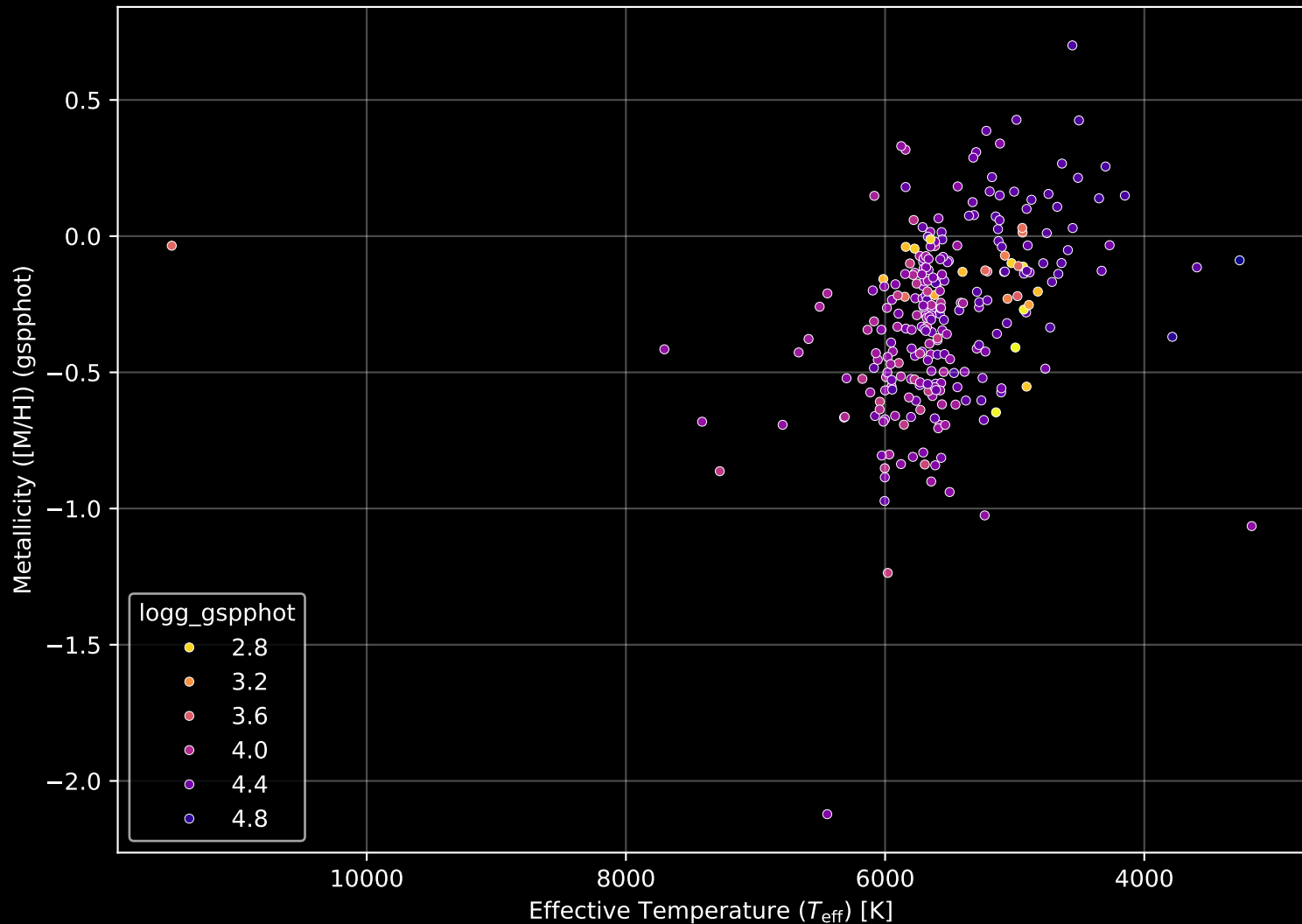
GALAH DR4 Field: [6957] Stellar Population Parameters (n= 268)
